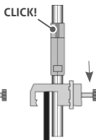
Ganci per pre-fissaggio
