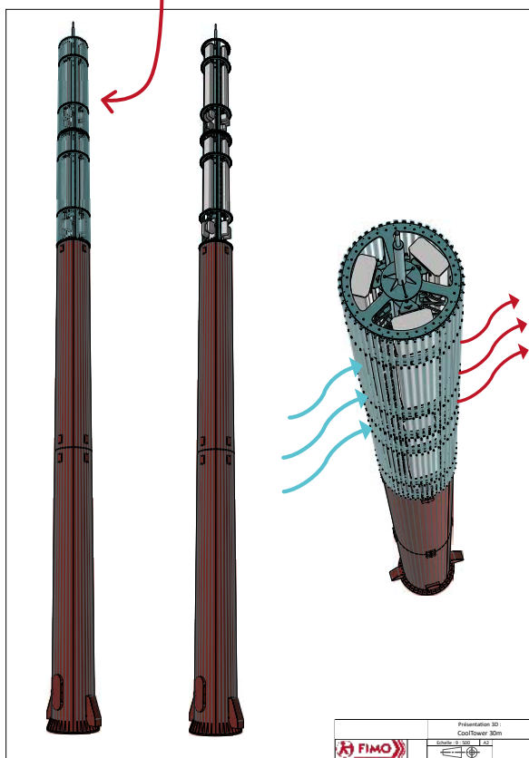
Pylône COOLTOWER®
